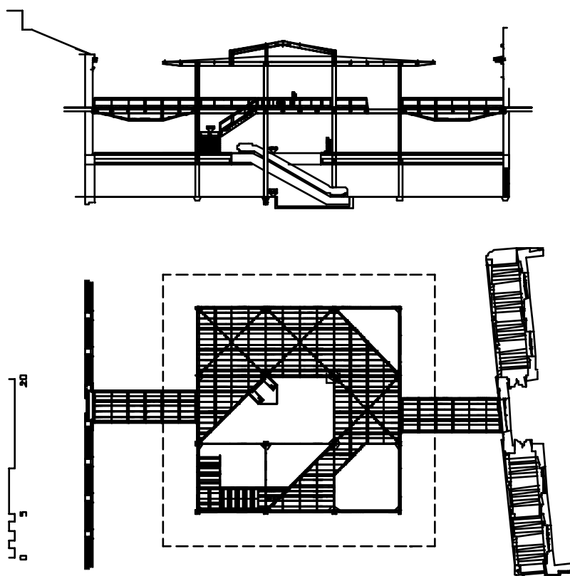
Planta piso y sección accesos.
